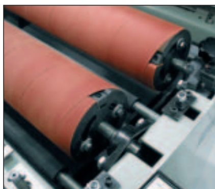
2 Schleifrollen für Grob- und Feinschliff in einem Arbeitsgang
