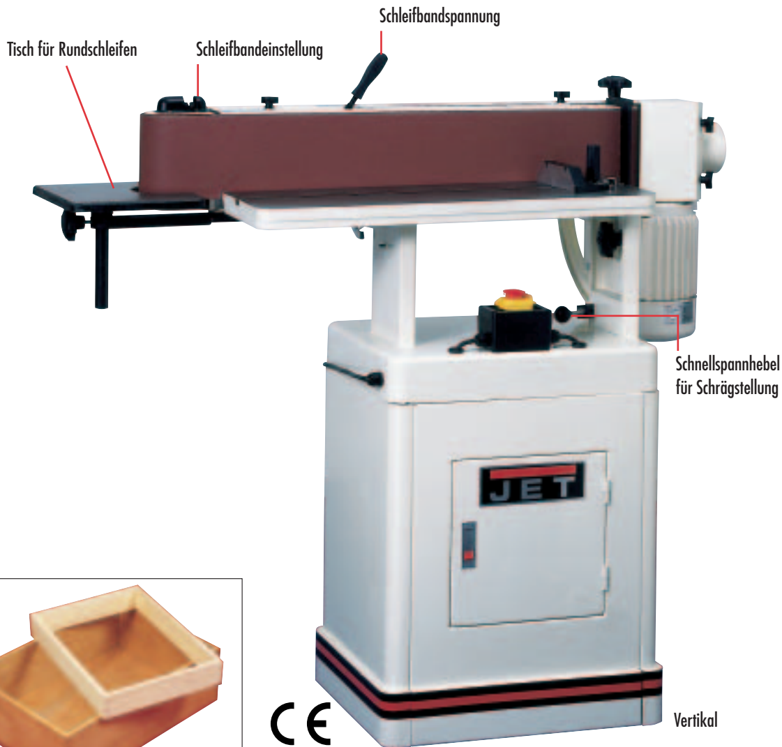
Schleifen von Schubladen mit dem Bandschleifer
